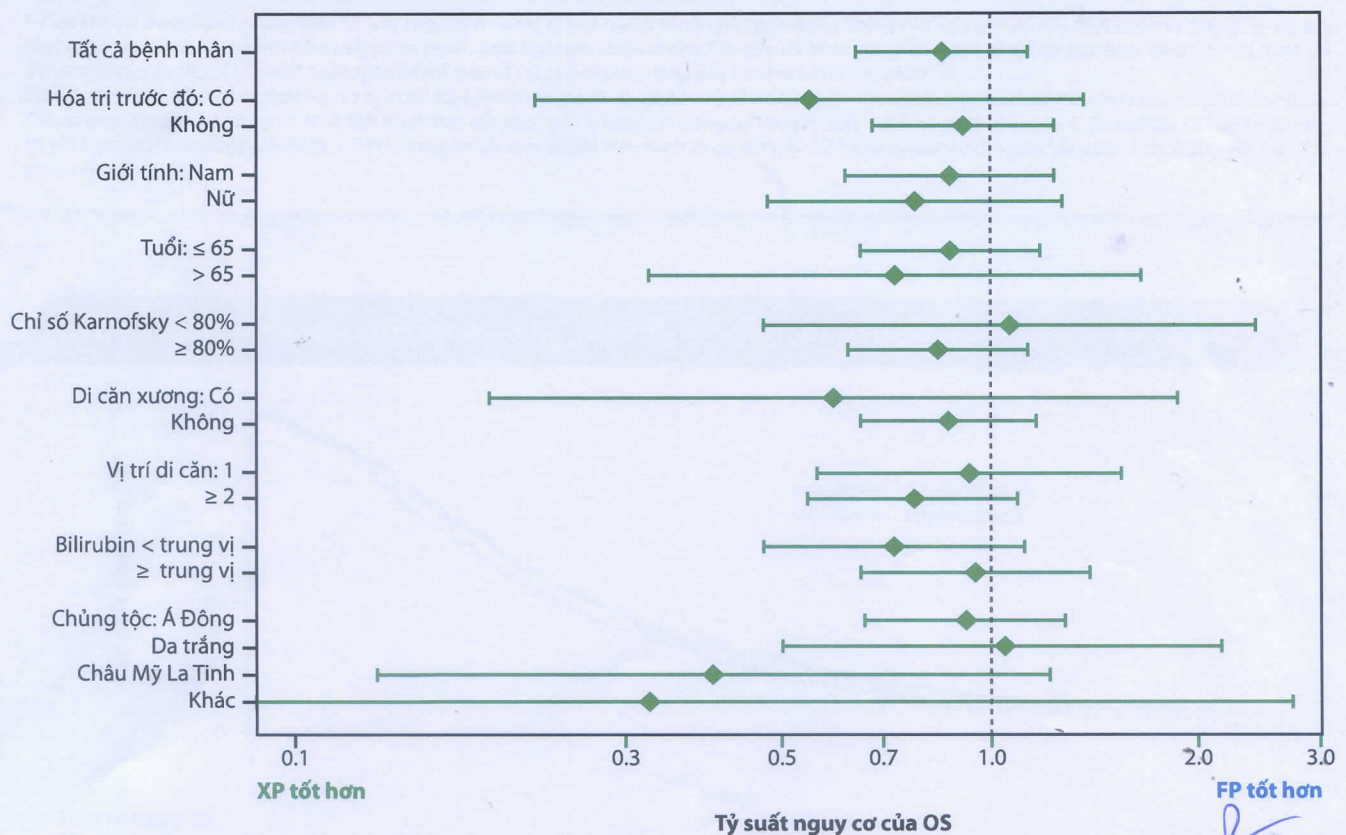
Bảng phân tích tỷ suất nguy cơ của các phân nhóm bệnh nhân tham gia nghiên cứu
