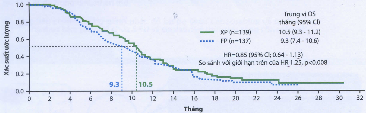
Biểu đồ Thời gian sống còn toàn bộ (OS)
